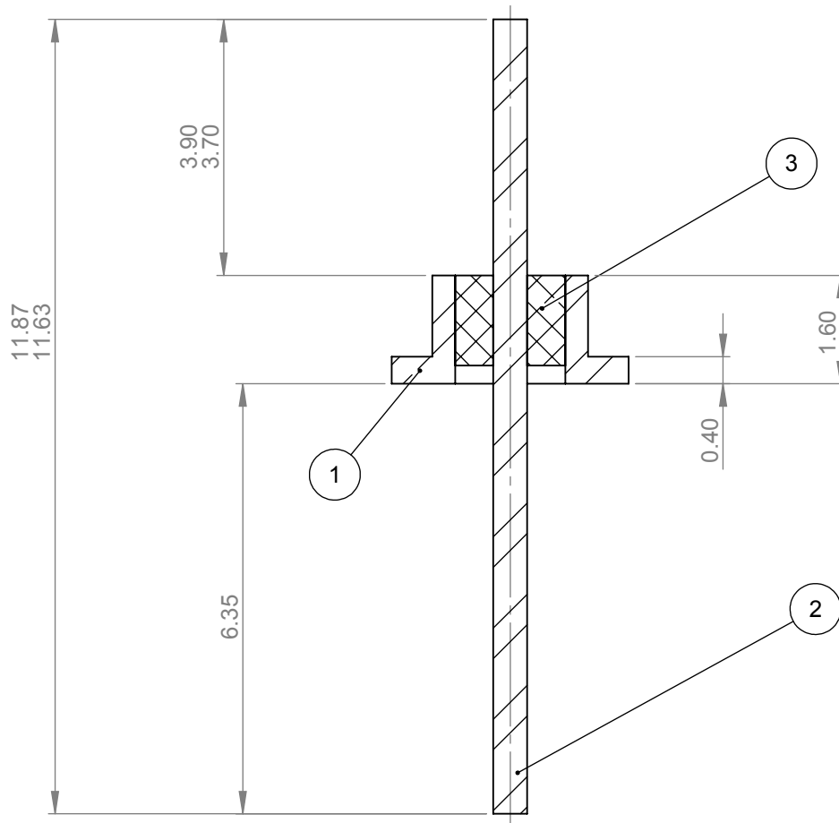
SECTION A-A
