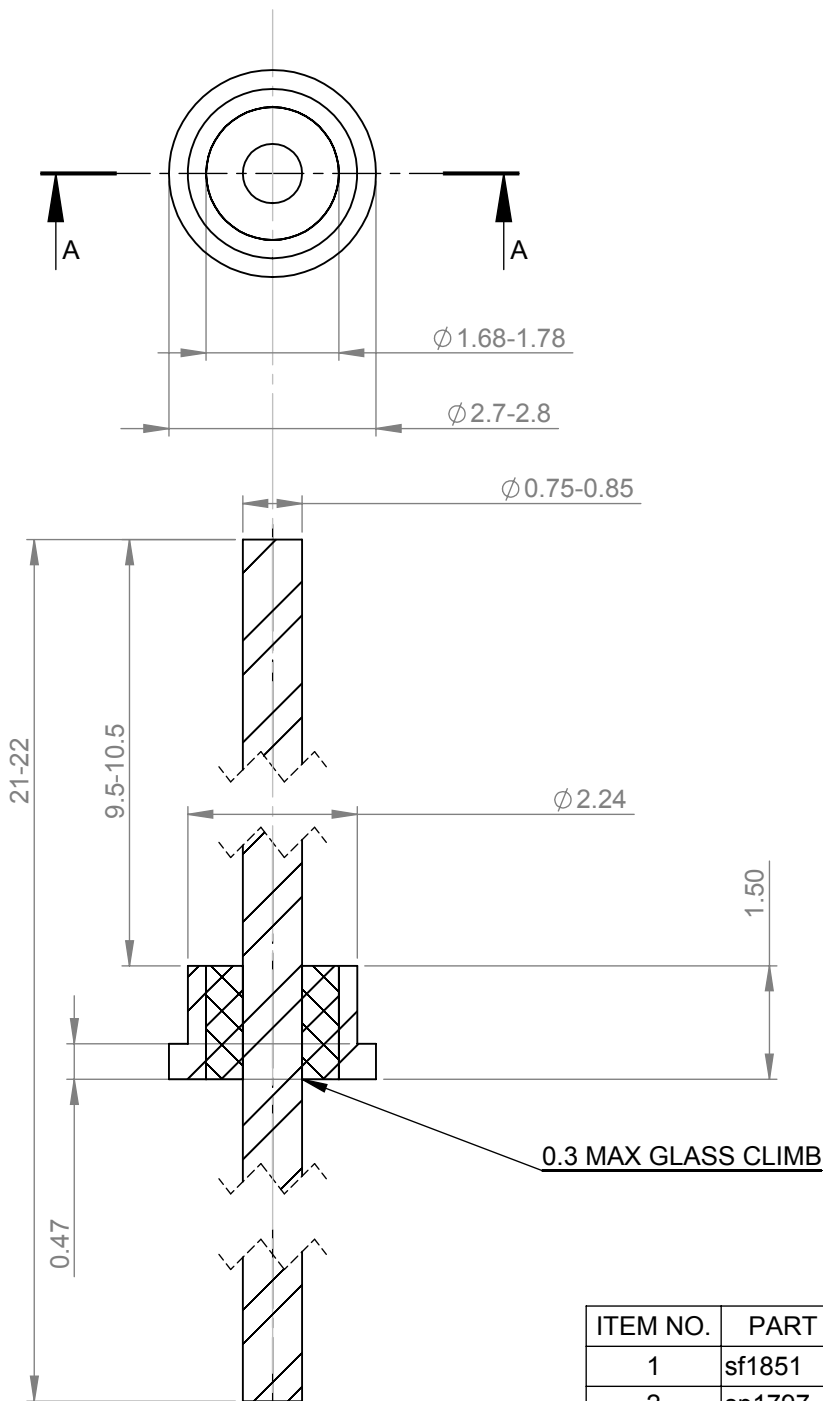
SECTION A-A SCALE 10 : 1
